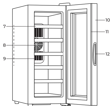
Вид изнутри
